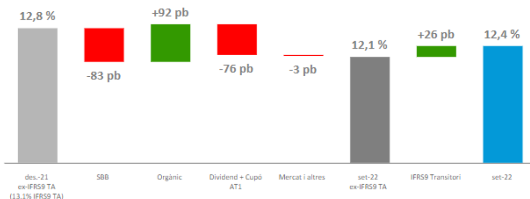
Evolució CET1
